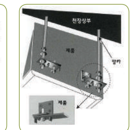
브라켓 설치도면
